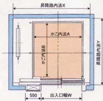
●昇降路平面図（サイドカウンター式）
