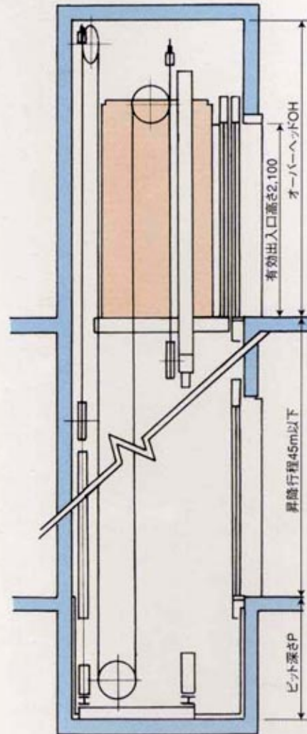
●昇降路断面図
