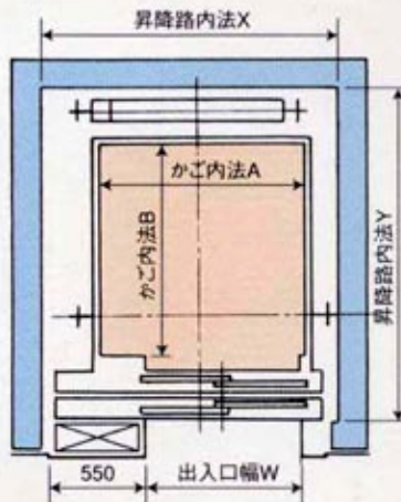
●昇降路平面図（バックカウンター式）
