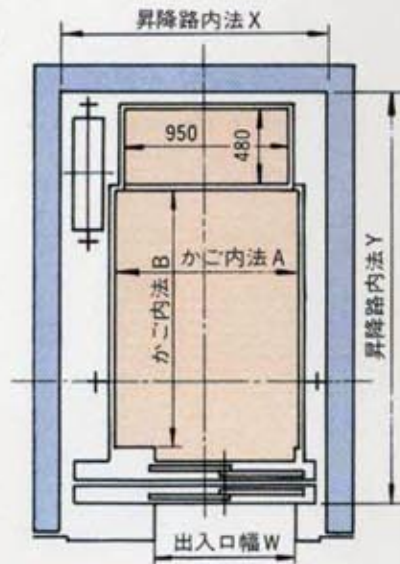
●昇降路平面図 (トランク付)
