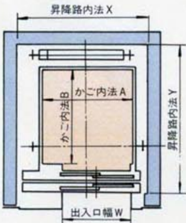
●昇降路平面図
